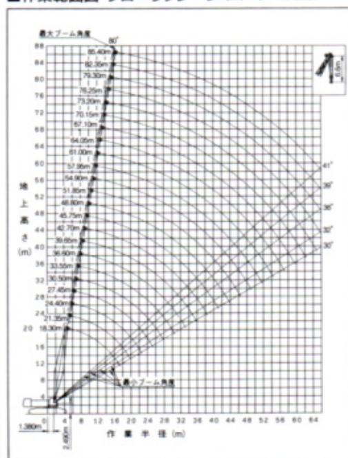
■作業範囲図 クローラクレーン (ロワーウェイト仕様)
