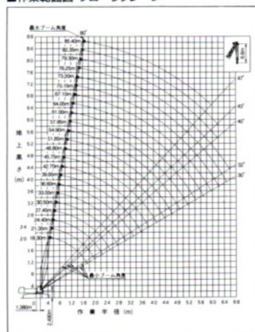
■作業範囲図 クローラクレーン
